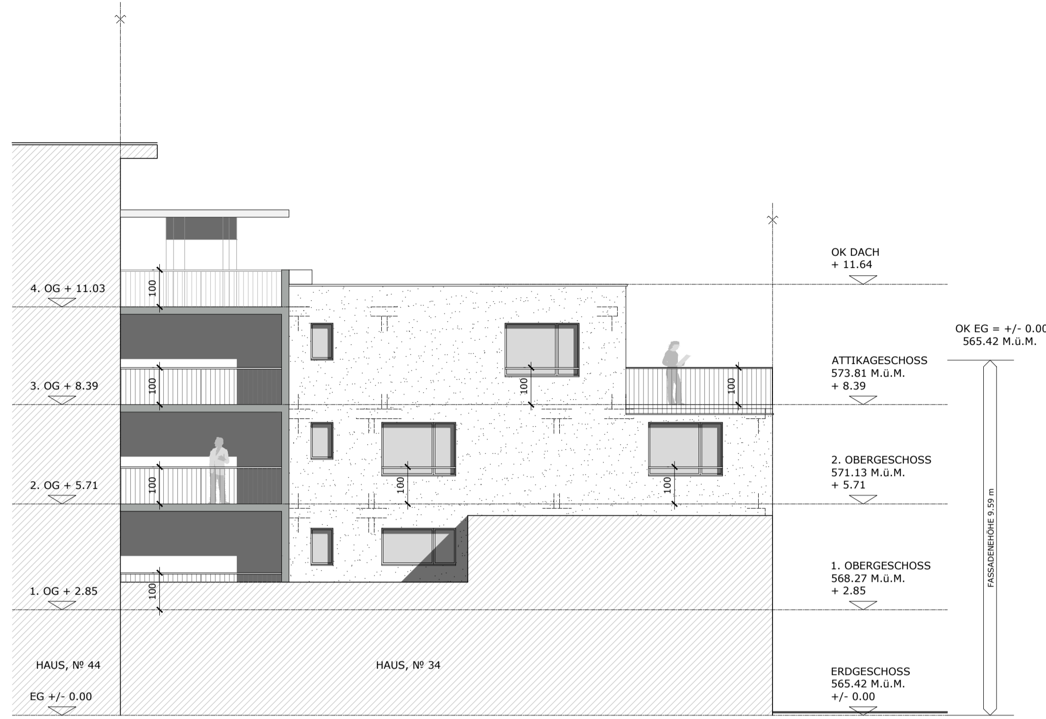
SÜDFASSADE
