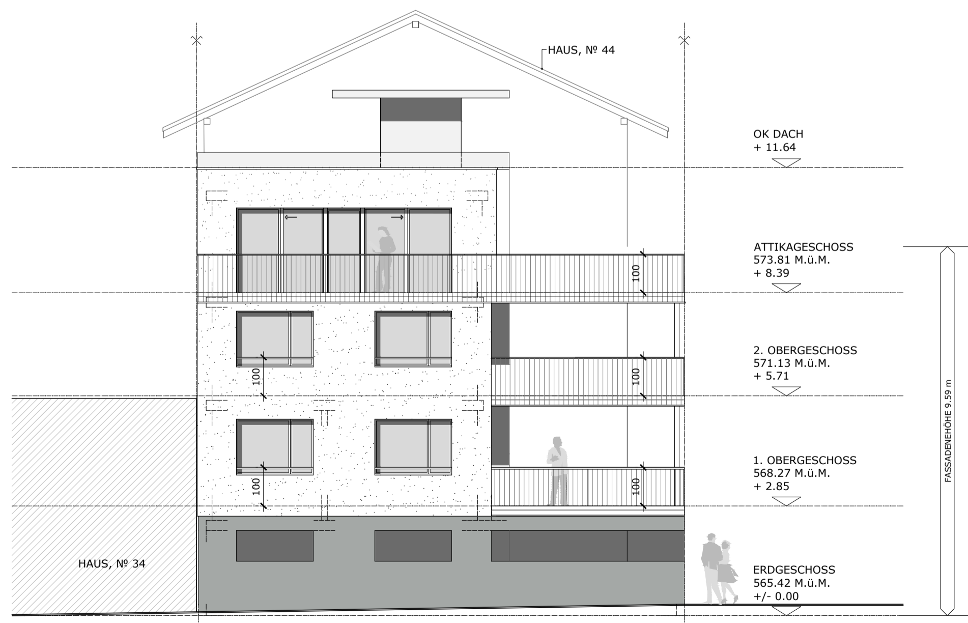
OSTFASSADE
