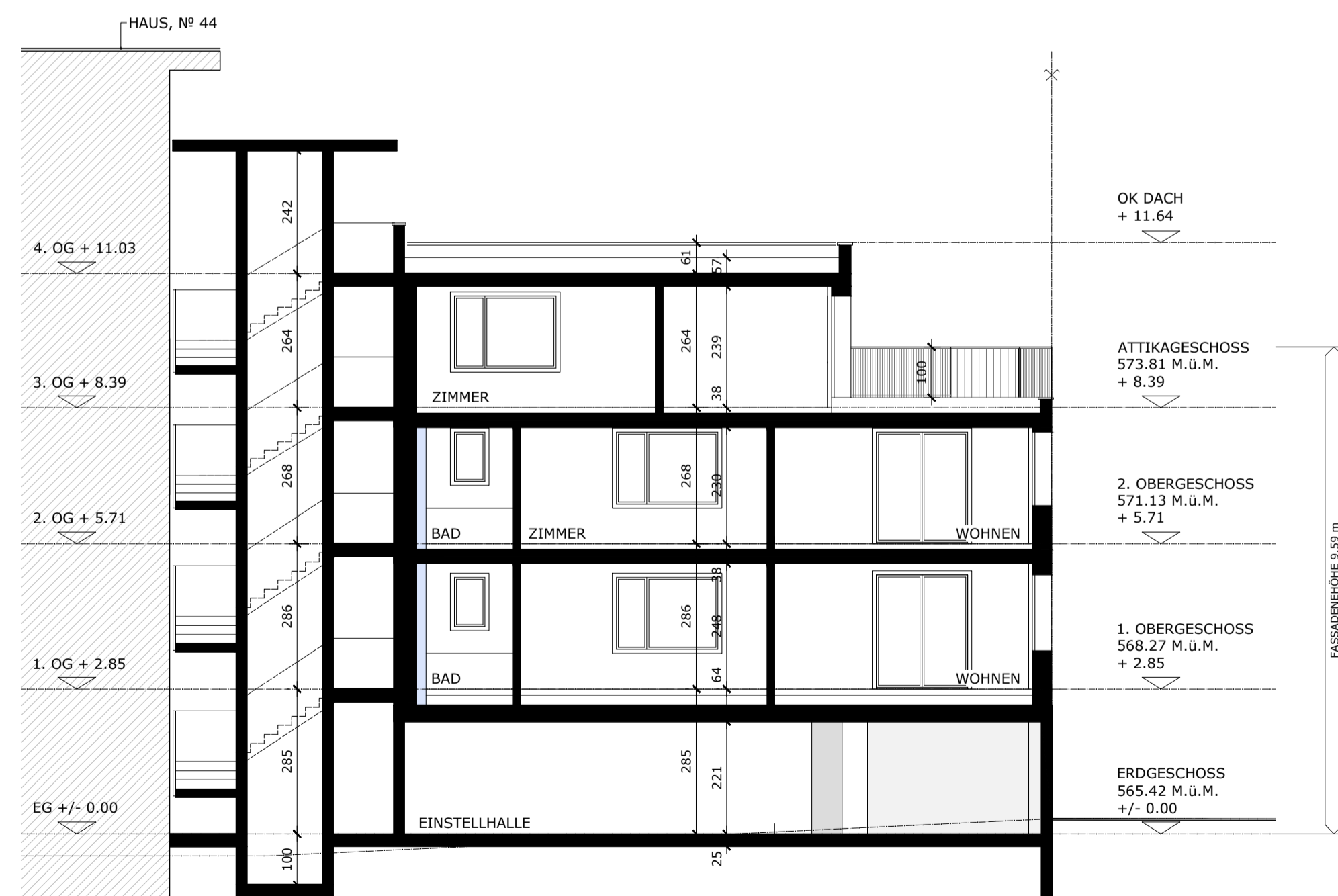
SCHNITT A-A
