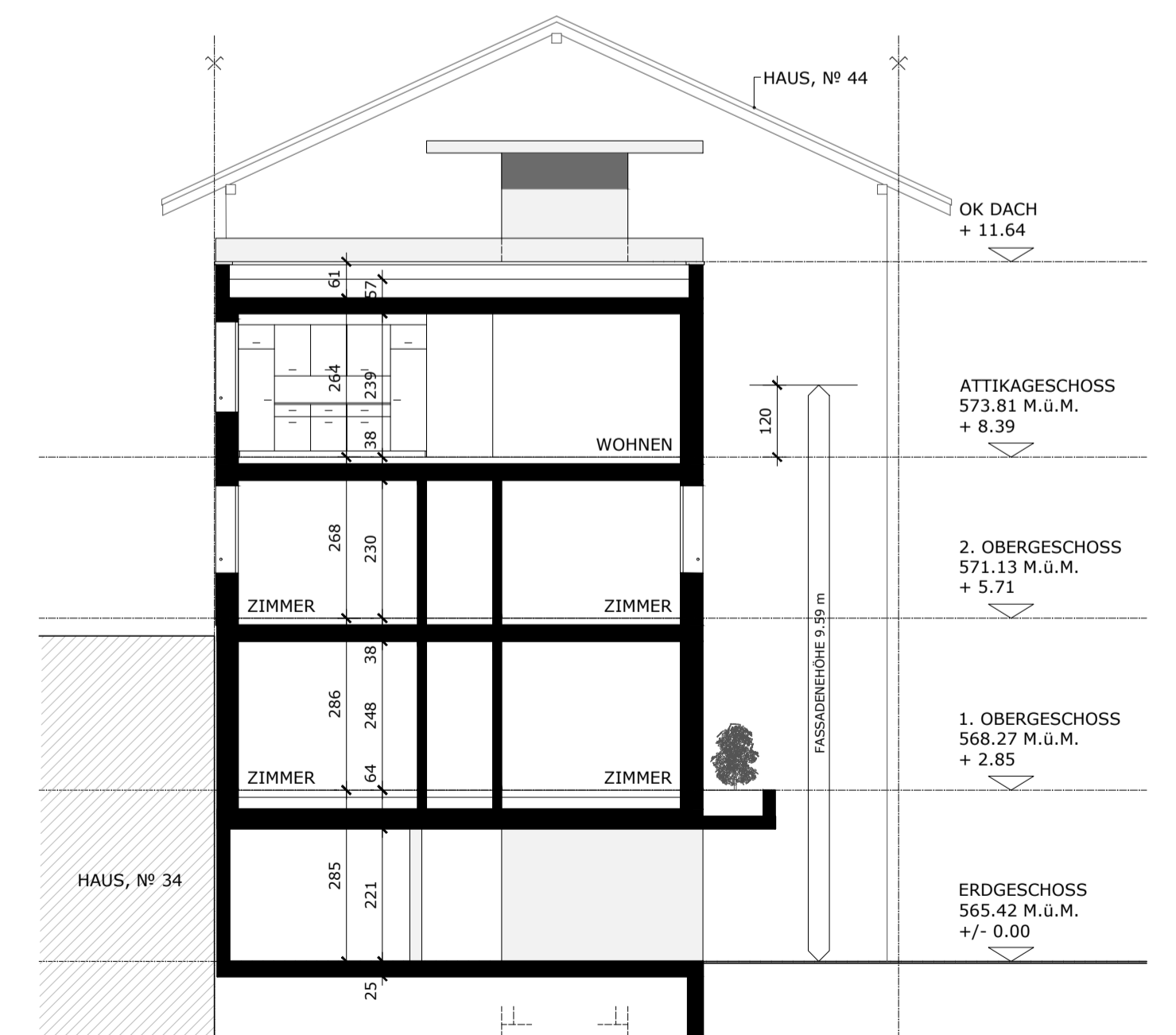
SCHNITT B-B
